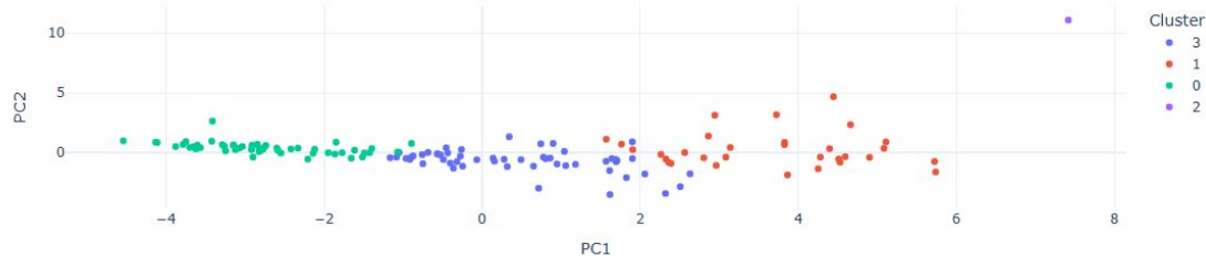
Clusters de pays (K-means=4) dans le plan ACP (PC1-PC2)
